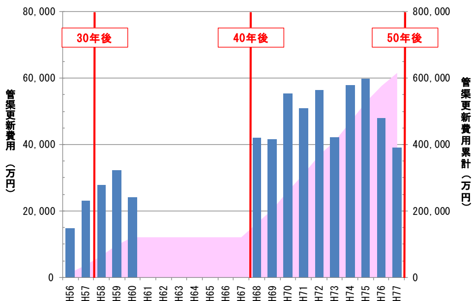
図-2.4.4 下水道管渠の年度別更新費用
