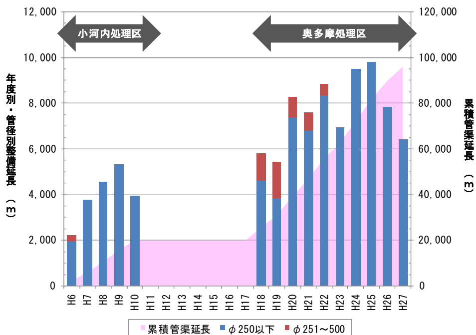
図-2.1.18 下水道管渠の年度別・管径別整備延長 (平成27年度は工事実績より推定)
